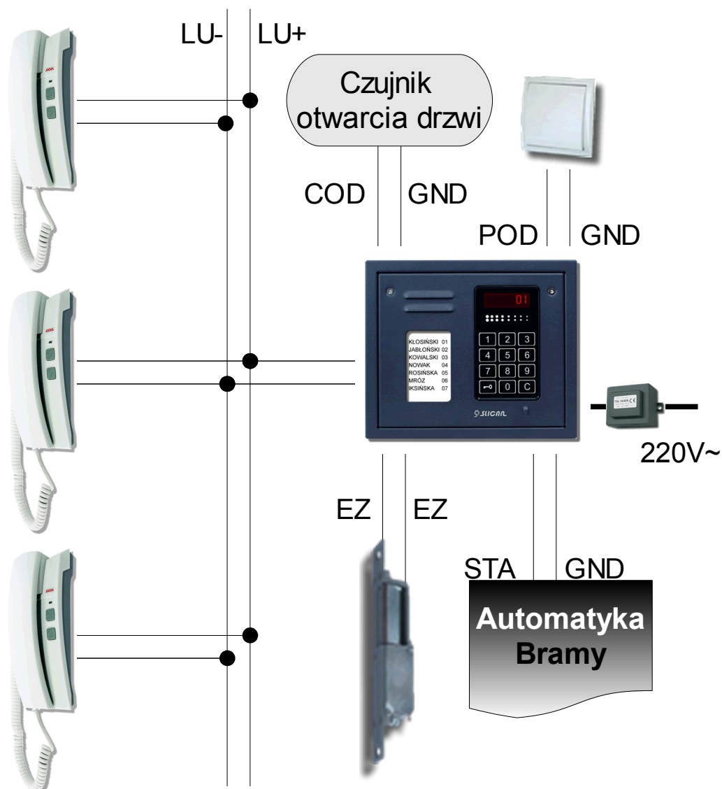
Ilustracja 2.2.: Magistrala unifonów
